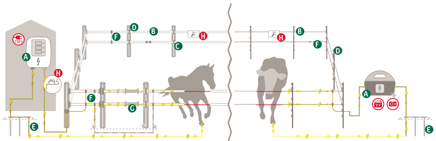
Permanentzaun mit 230 Volt Versorgungsspannung
