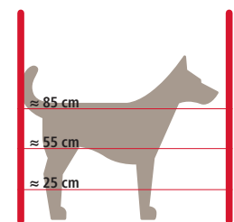
Elektrozaun für große Hunde Empfehlung: Hobbyset, Litze
